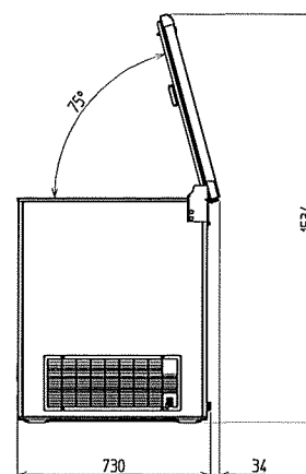
扉開閉図(1:15)
