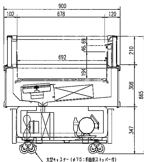
機械室レイアウト (X-SR-MG587/687BRA-K)
