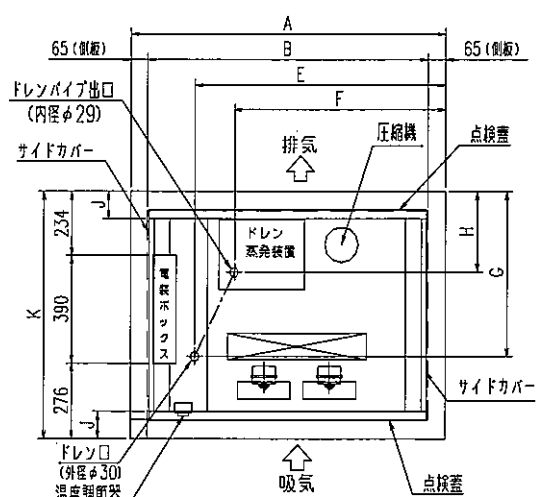
機械室レイアウト (X-SR-MG487BRA-K)
