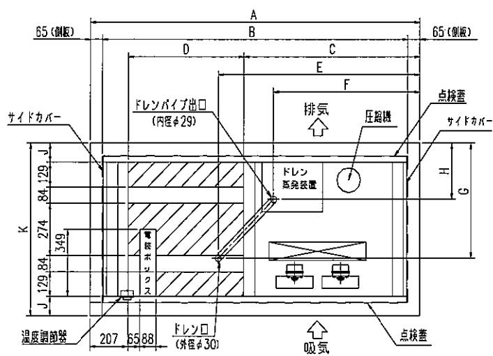
機械室レイアウト (X-SR-MG587/687BRA-K)
