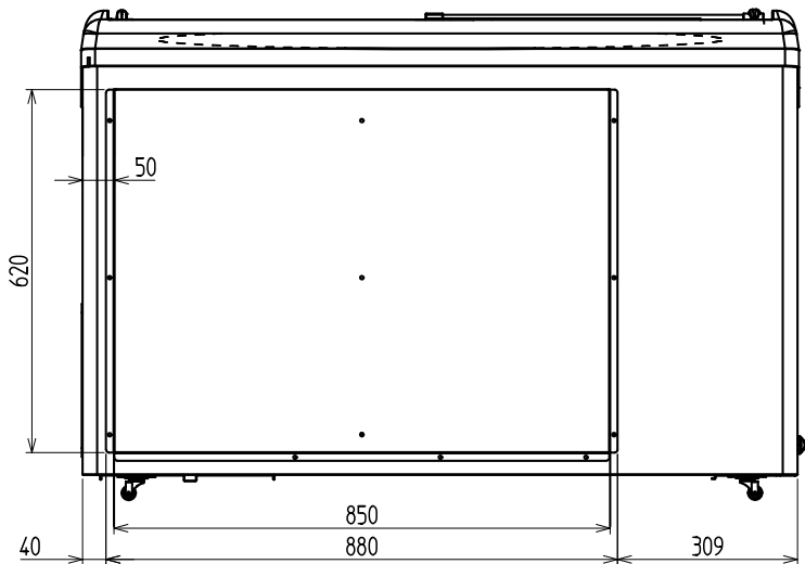
矢視A
