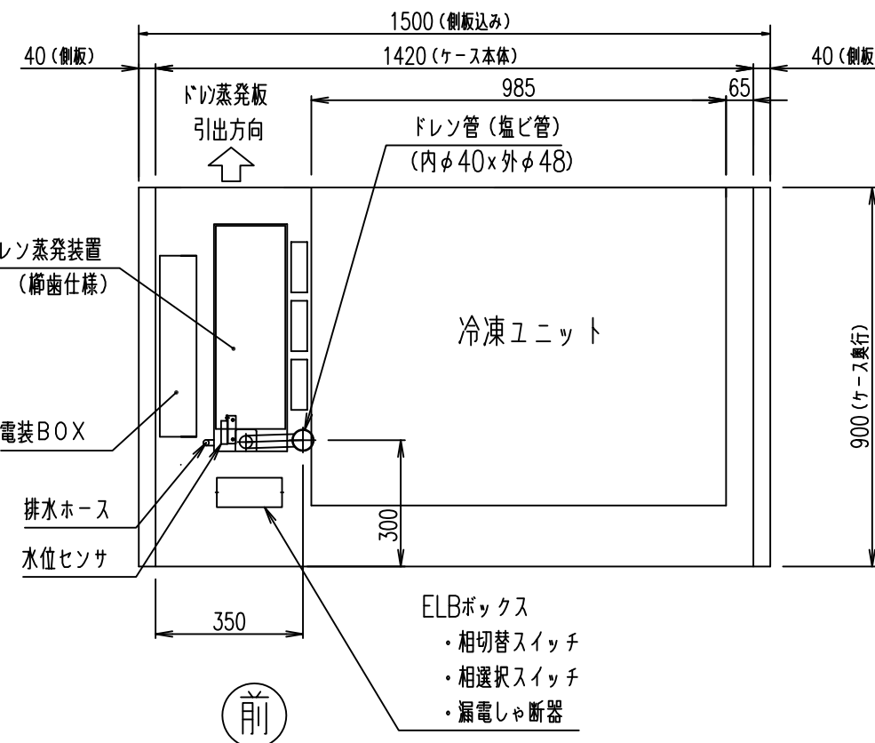
機械室内レイアウト
